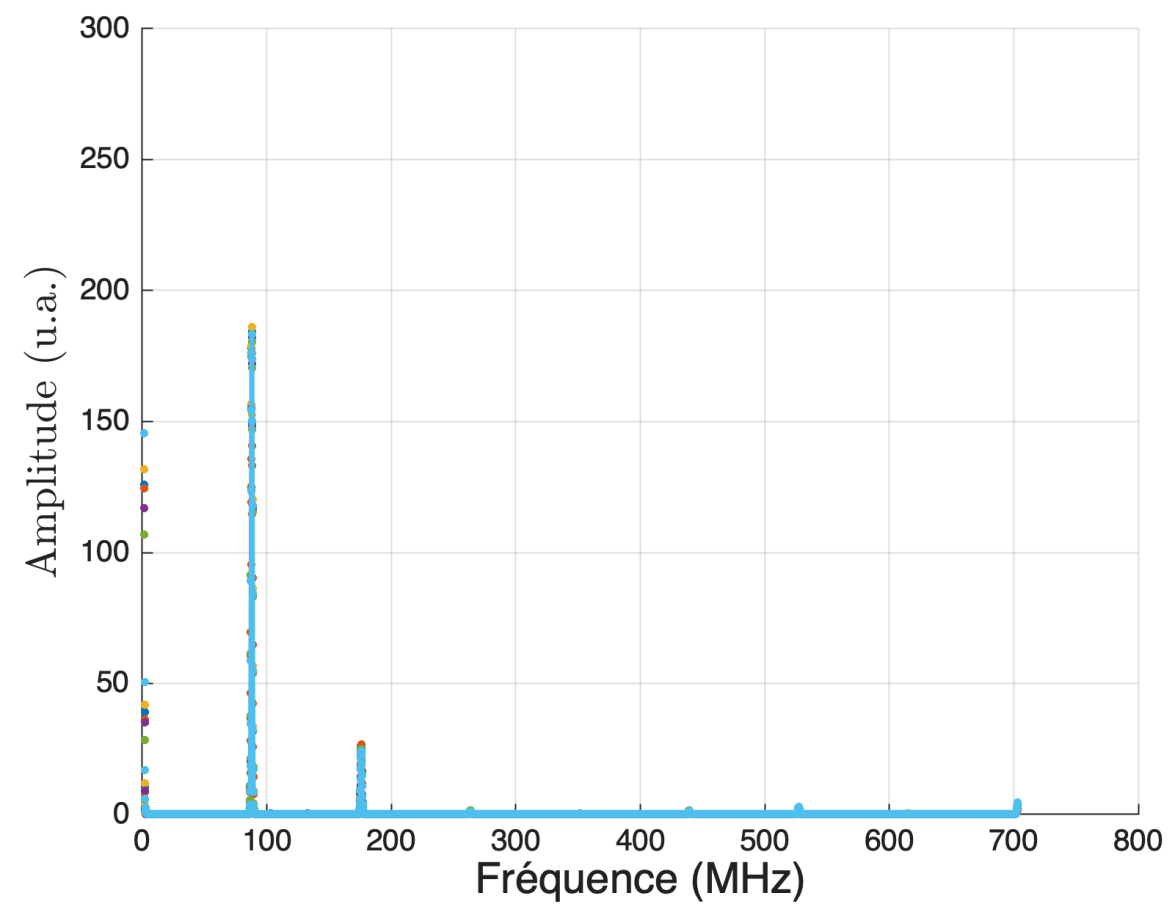
FIGURE 27 – DSP totale résultant d’une mesure faible temporelle. Ici, les lignes verticales représentent la position des pics de puissance dans le spectre. La fréquence centrale est de 703,12\text{ MHz} pour une durée spectrale de 1,4062\text{ GHz} avec une résolution temporelle de 4\text{ ps} . La figure 28 montre un zoom sur le pic de puissance à 175,8\text{ MHz} .
