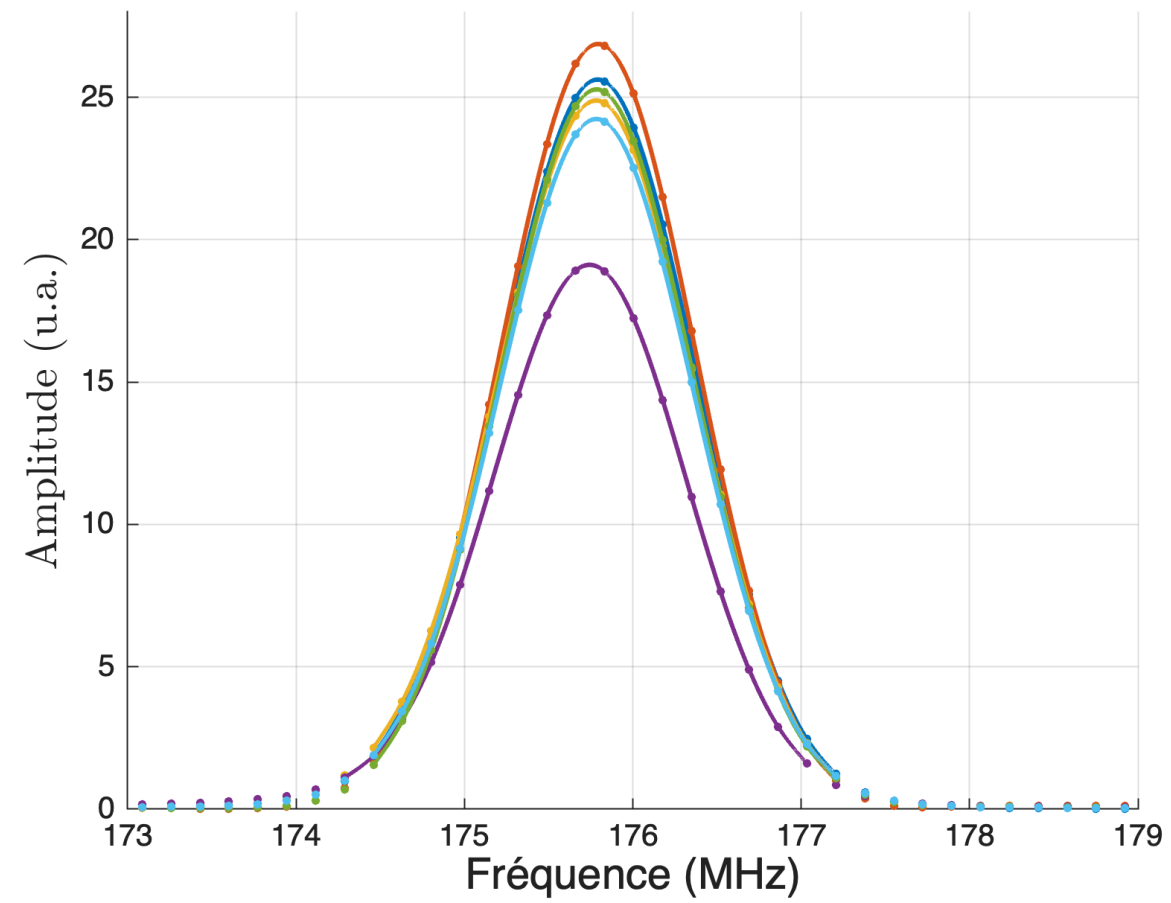
FIGURE 28 – Zoom sur le pic de puissance à 175,8\text{ MHz} . On peut observer la présence de plusieurs pics de puissance, avec leur ajustements paramétriques polynomiales du quatrième ordre pour déterminer chaque position fréquentielle des états d'entrée.
