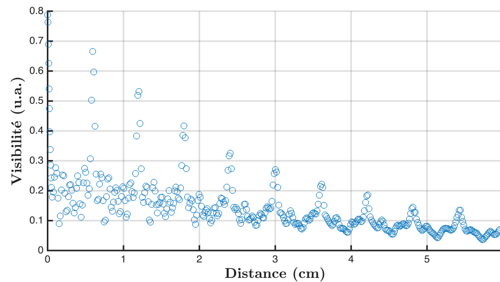
FIGURE 16 – Spectre de visibilité de notre laser. La visibilité obtenue est d'environ 0,7877. On constate que le pic de visibilité à 0 cm correspond à l'état de polarisation verticale |V\rangle , tandis que le pic à 1,2039 cm correspond à l'état de polarisation horizontale |H\rangle avec une visibilité de 0,5318 . Le pic à 0,5943 cm est dû à l'état de superposition donc à l'interférence entre les deux états de polarisation, avec une visibilité de 0,6654.
