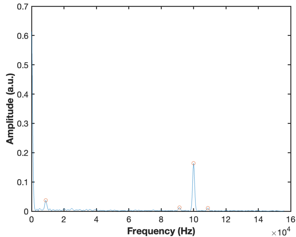
FIGURE 31 – Ensemble du spectre obtenu de l'oscilloscope pendant l'effet Doppler
